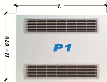
Dimensioni nicchia (per installazione senza FDI) - Nike dimensions (for installation without FDI) (Ln) x (Hn = 620) x (Sn = 220)
