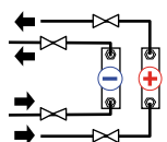
4 TUBI (2 batterie) 4 PIPE (2 coils)
